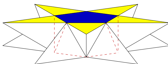
（圖 b）五角星形源自正二十面體凸出角錐的三角面（淺色）恰與反五角柱的五邊形（深色）共平面。
