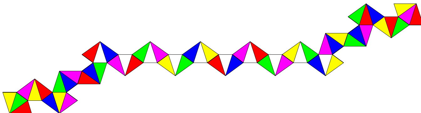
（圖 c）二十星體一體成型的展開圖（同色的 10 個三角形將組成 2 個互相平行的五角星）。
