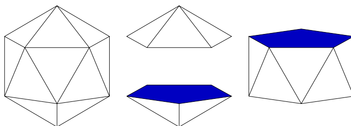
（圖 a）正二十面體（左）可分解成 2 個五角錐（中）和 1 個「反五角柱」（右）。
